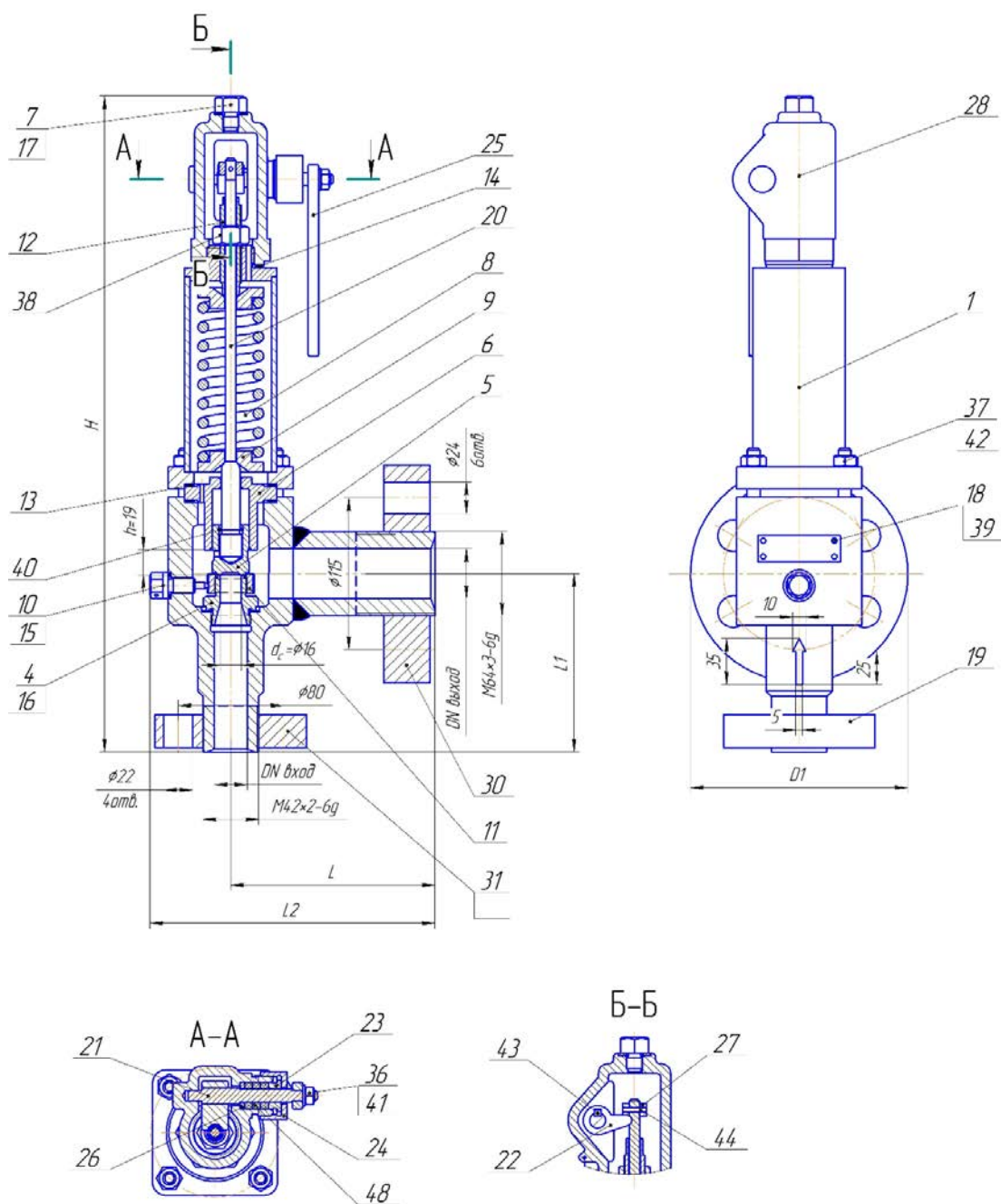
Чертеж общего вида (вариант 2)
